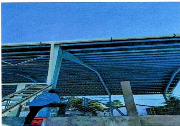
Foto1: COLOCACIÓN DE CANALES PARA CAIDAS PLUVIALES
